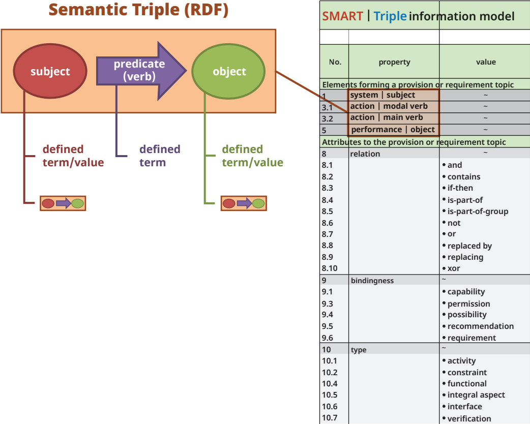
Abbildung 40: Triple-Strukturierung für zukünftige Entwicklungsprozesse unter Nutzung des Informationsmodells
