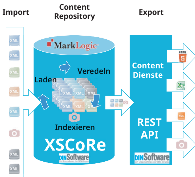
Abbildung 32: Überführung des DIN-Normenbestands in XML
