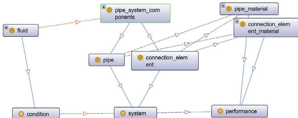
Abbildung 43: Automatisierte Übersetzung in OWL/RDF
